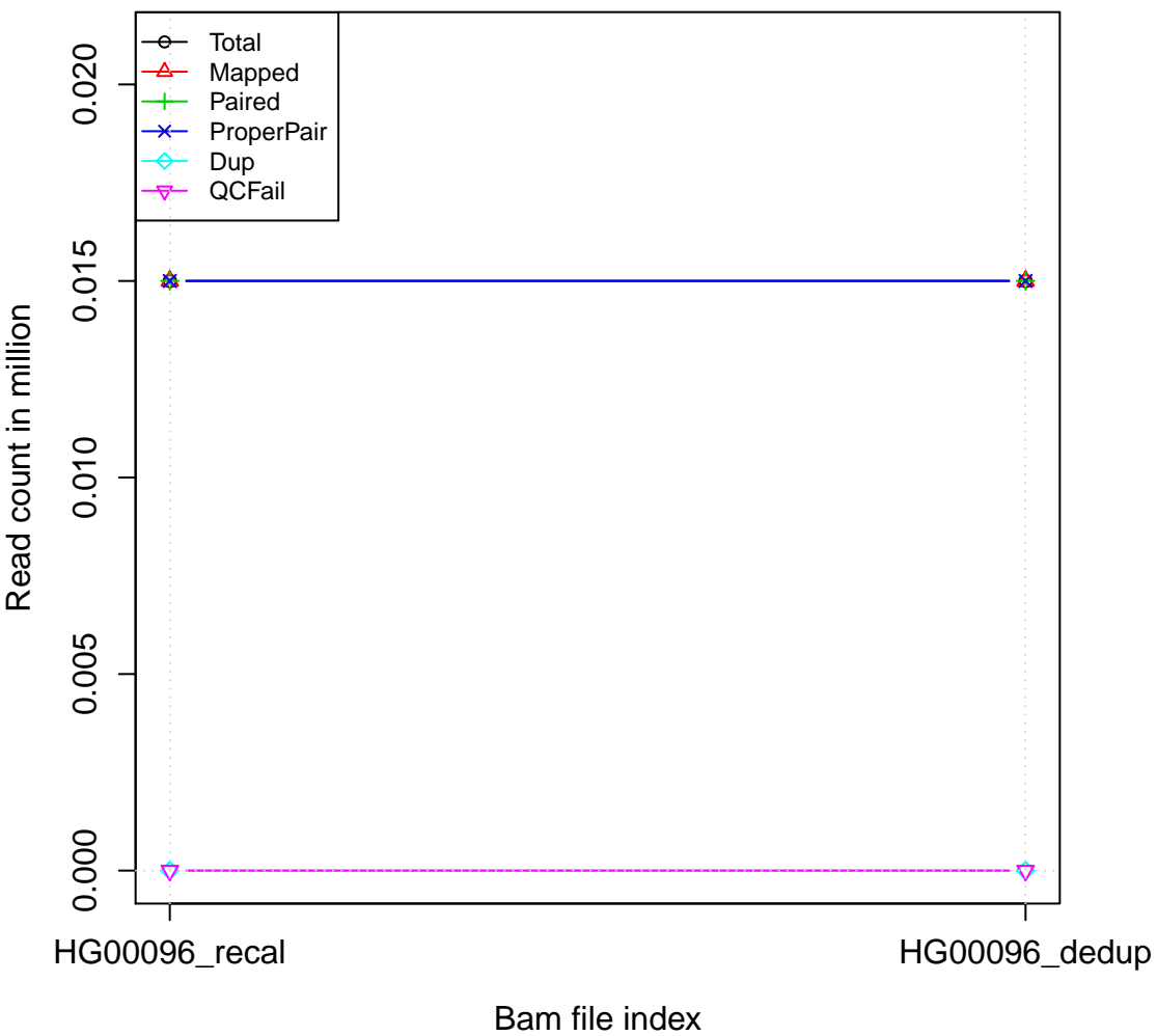
Flag stats
