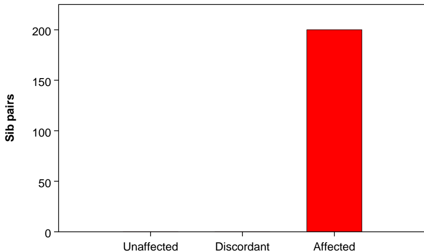
Sib pairs
